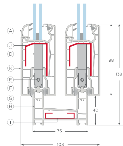
CORTE PUERTA NEW S75/98 DOBLE RIEL
