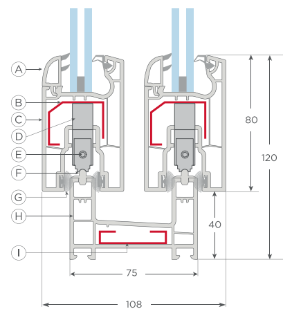
CORTE VENTANA NEW S75/80 DOBLE RIEL
