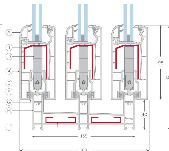
CORTE PUERTA NEW S75/98 TRIPLE RIEL
